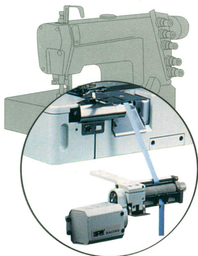
MC S6B-57 下送用 FROM BOTTOM FEED
