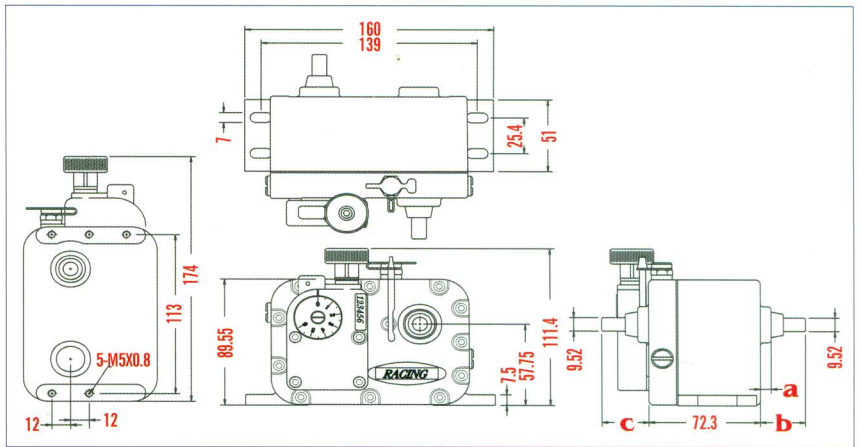
尺寸圖 Specification
