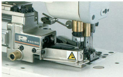
TCM-M45/C
